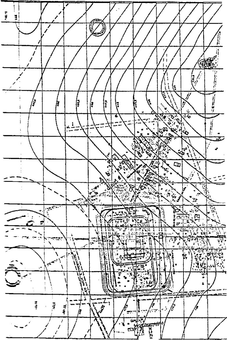
Abb. 3. Zugmantel, Kastell und Kastellvicus. Übersichtsplan mit rekonstruiertem Strassennetz M. 1:4000. Sommer 1988, Abb. 5.
